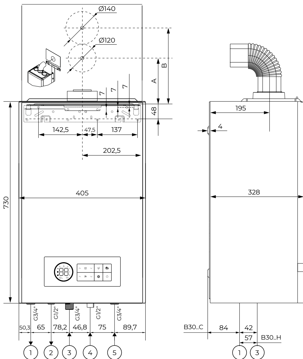
Рис. 28. V30 28 C/H, V30 32 C/H, V30 36 C/H.
